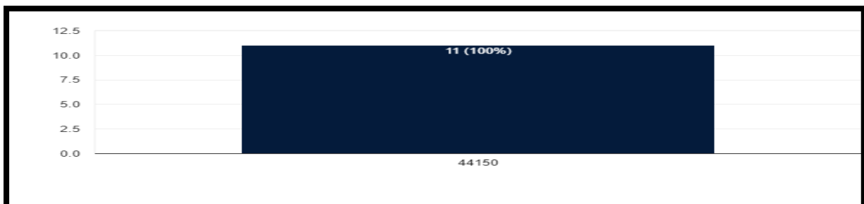
Figura 7: Código postal.
